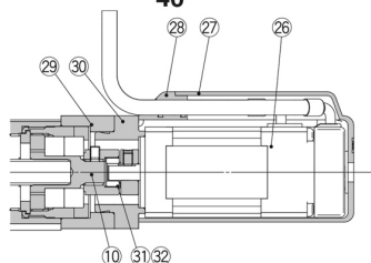
Axialer Motor: LEY 16 25 32 40 D
