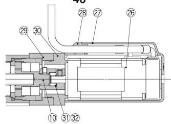
Axialer Motor: LEY D 16 25 32 40
