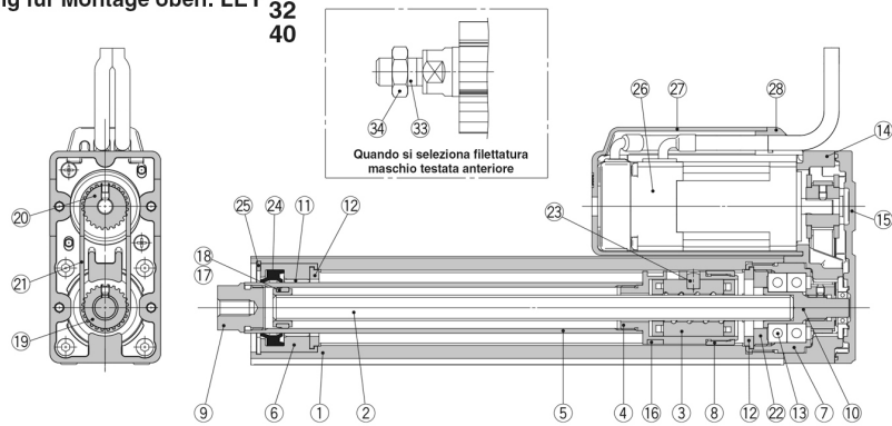
Motorausführung oben/parallel Mit Verriegelung/Motorgehäuse
