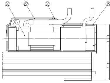
Axialer Motor: LEY 16 25 32 40 D
