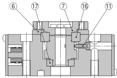
Modèle standard
