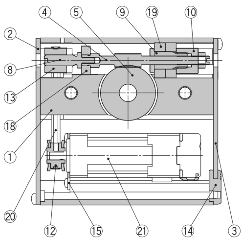
Modèle standard
