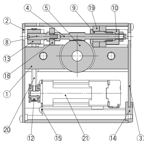
Modèle standard
