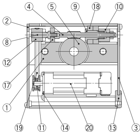
Präzisionsausführung
