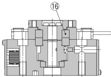
Präzisionsausführung
