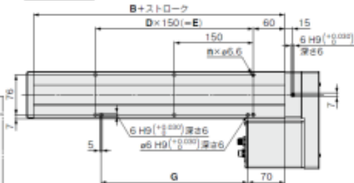
寸法表
