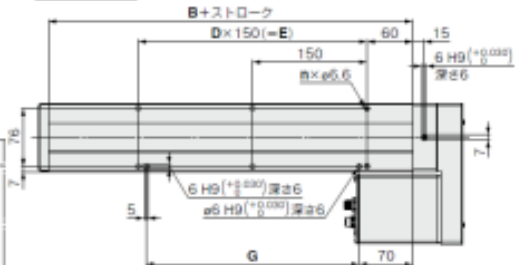
寸法表
