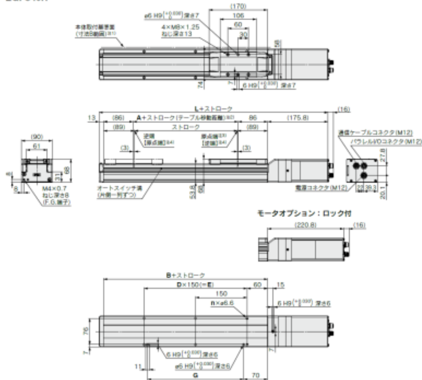
寸法表
