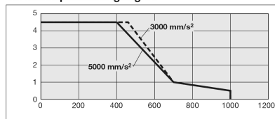
Vertikal/Spindelsteigung 30
