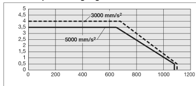
Vertikal/Spindelsteigung 24
