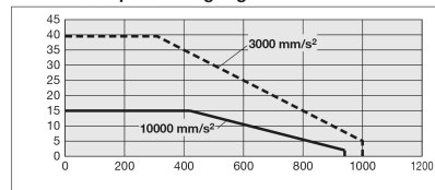
Vertikal/Spindelsteigung 24
