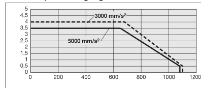
Vertikal/Spindelsteigung 24
