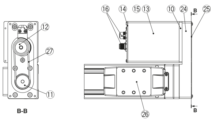
Parallele Motorausführung für Montage rechts/links
