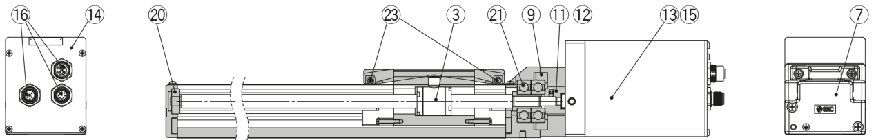
Axialer Motor
