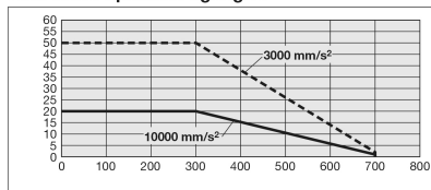
Vertikal/Spindelsteigung 16
