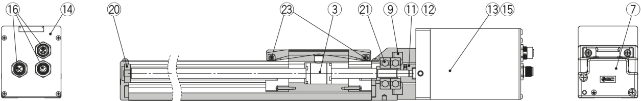
Axialer Motor
