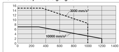
Vertikal/Spindelsteigung 20
