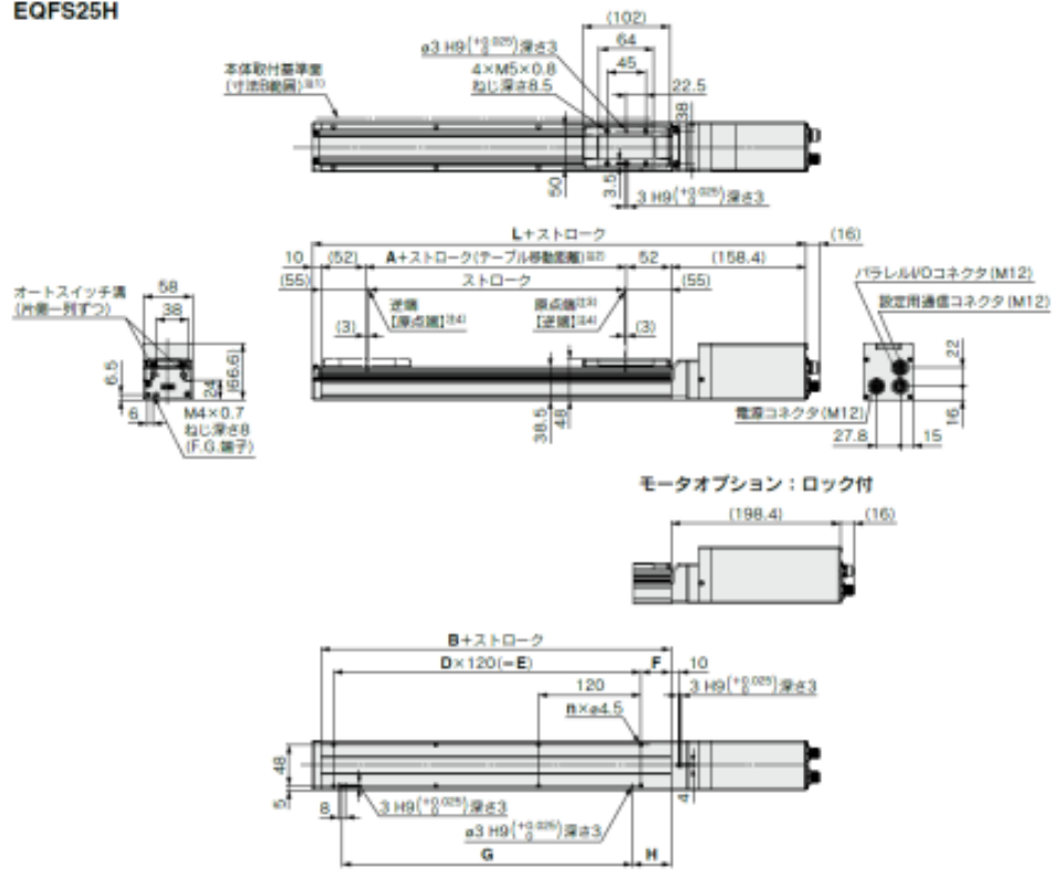
寸法表
