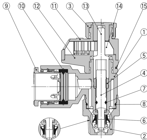
zuluftgesteuert abluftegesteuert
